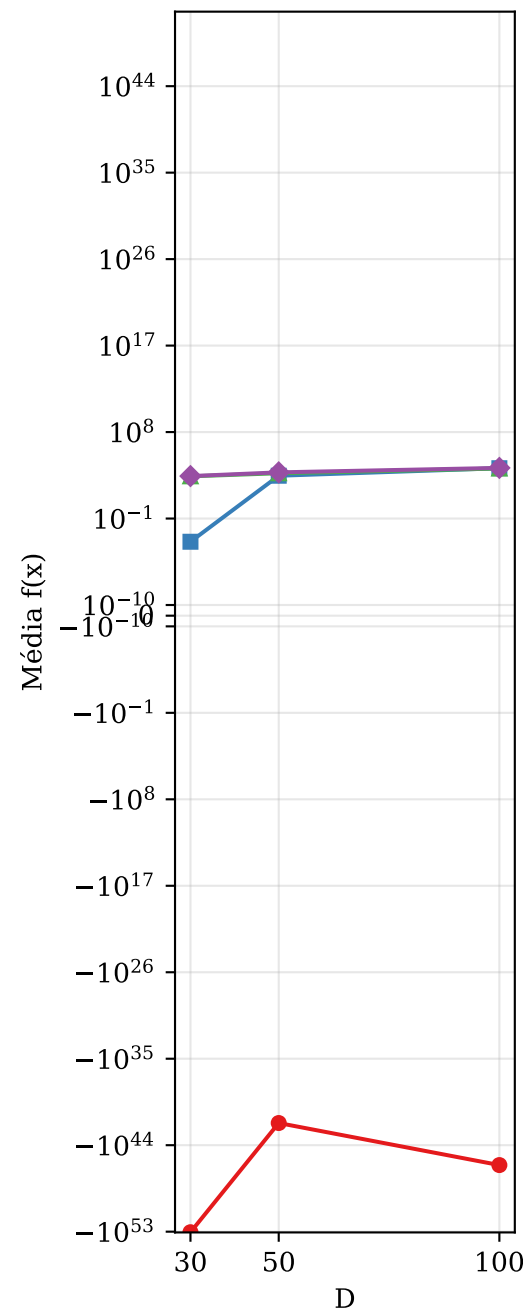
Schwefel 2.26
