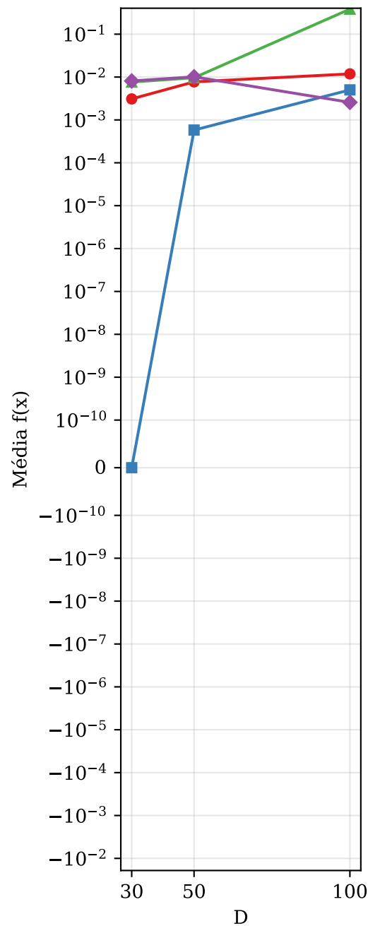
Griewank
