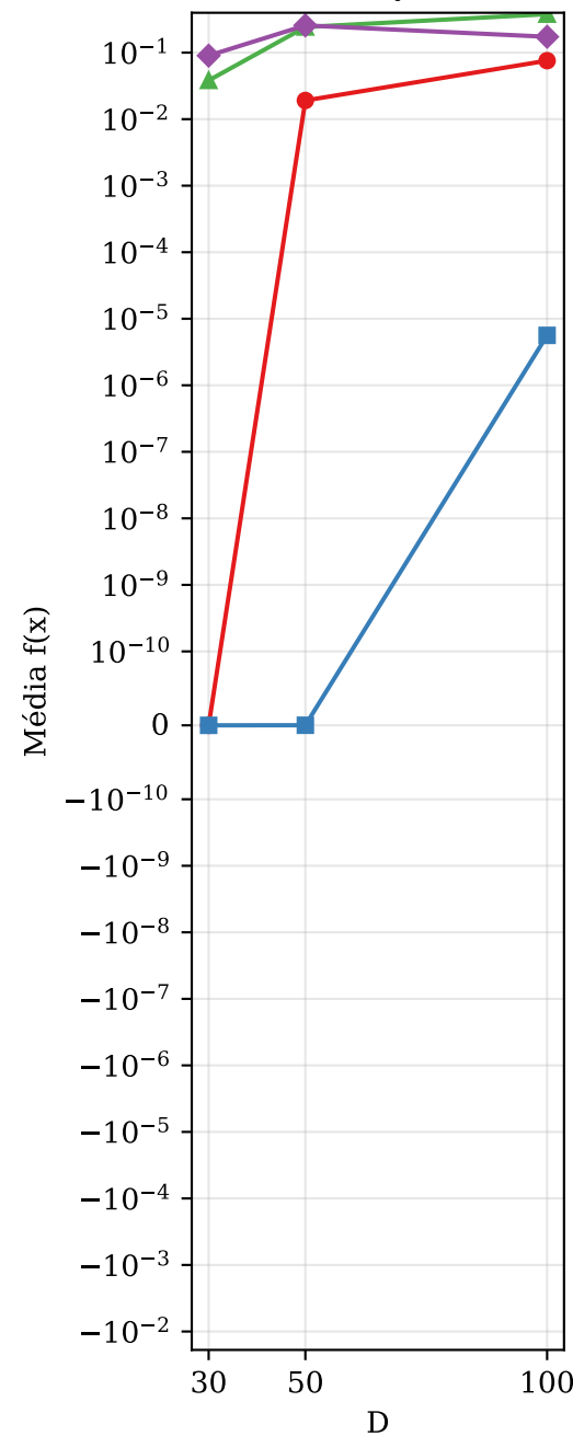
Lévy
